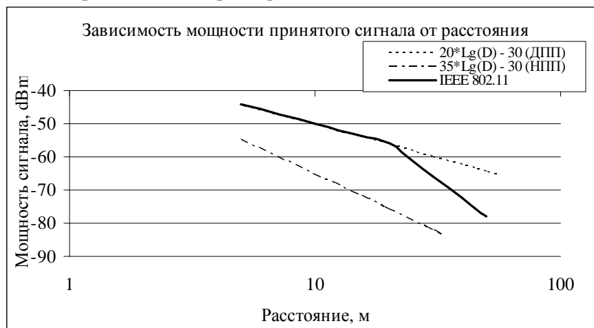
Рис. 8. Сравнение модели IEEE 802.11 с ДПП и НПП каналов Fig. 8. IEEE 802.11 channel model comparison with UDP and DDP channel models
