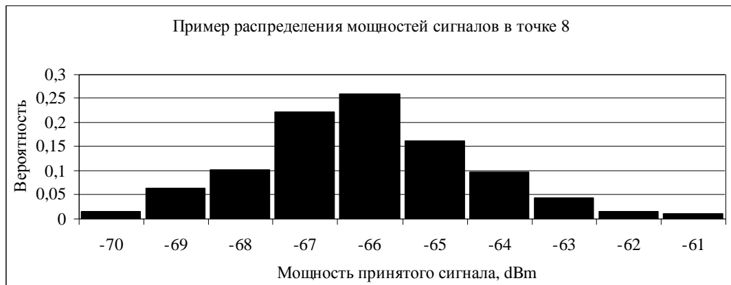
Рис. 7. Статистическое распределение мощностей принятых сигналов для НПП канала Fig. 7. Received signal strength statistical distribution for UDP channel
