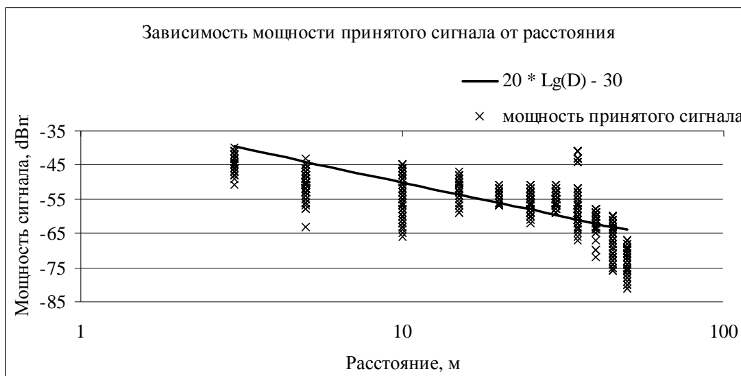
Рис. 4. Зависимость мощности принятого сигнала от расстояния для ДПП канала. Fig. 4. Received signal strength dependence from distance for DDP channel
