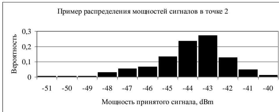
Рис. 5. Статистическое распределение мощностей принятых сигналов для ДПП канала Fig. 5. Received signal strength statistical distribution for DDP channel
