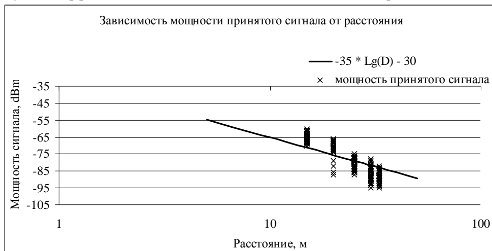
Рис. 6. Зависимость мощности принятого сигнала от расстояния для НПП канала Fig. 6. Received signal strength dependence from distance for UDP channel
