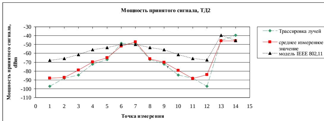
Рис. 4. Мощности принятых сигналов для точки доступа 2 (ТД2)
