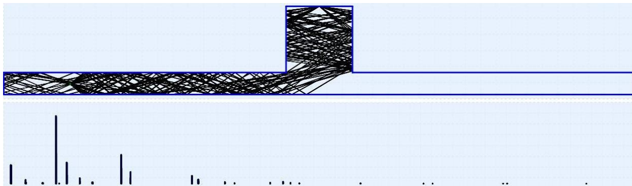
Рис. 1. Моделирование многолучевого канала в коридоре здания
