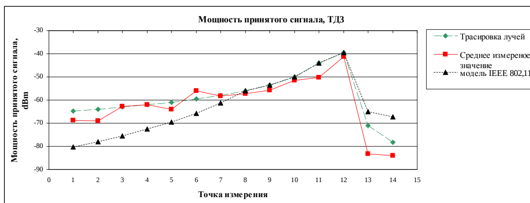
Рис. 5. Мощности принятых сигналов для точки доступа 3 (ТД3)
