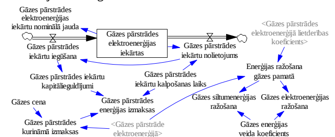
3. att. Koģenerācijas procesa apakšmodelis.
