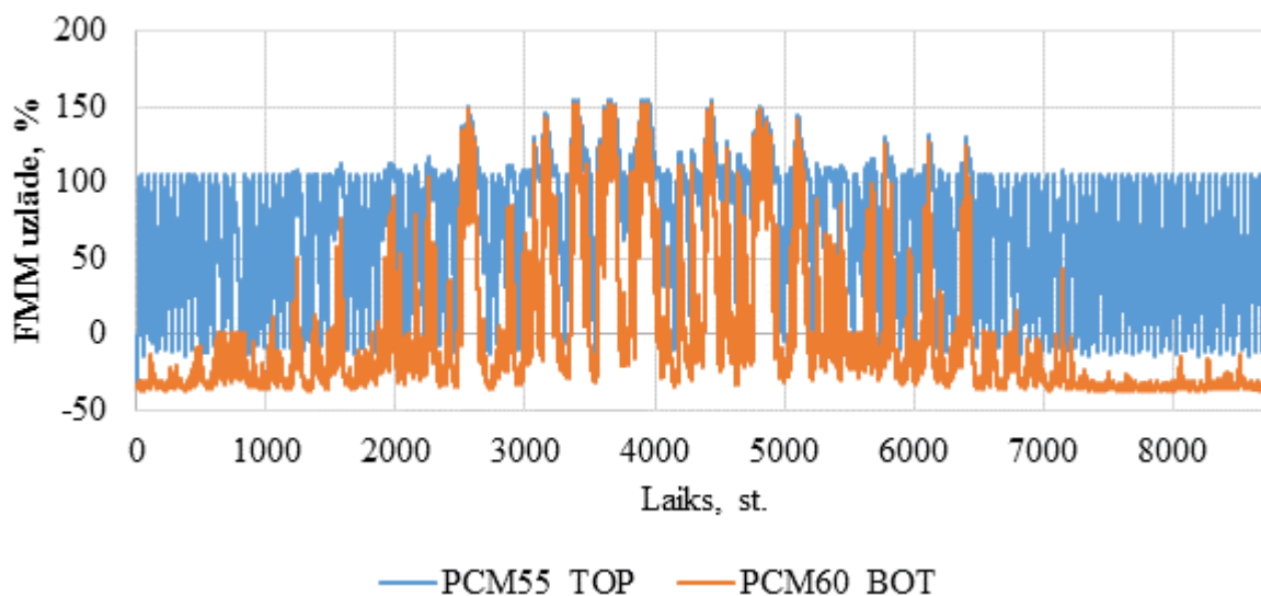
3.4. att. FMM uzlāde gada laikā divu FMM izkārtojumu ar 55 °C FMM augšpusē ( PCM55_TOP ) un 60 °C FMM ( PCM60_BOT ) apakšpusē.
