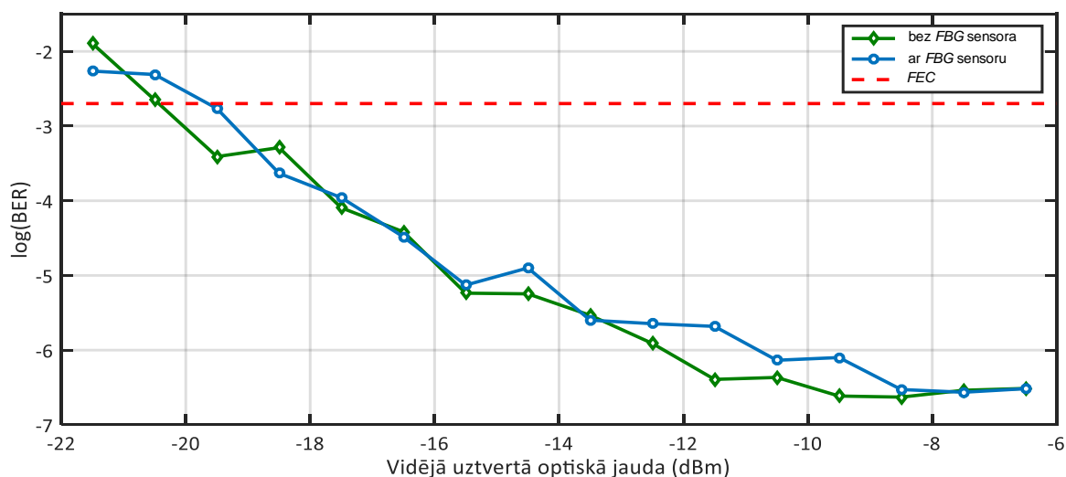
4.8. att. BER salīdzinājumā ar vidējo uztverto optisko jaudu 1,5 Gbit/s spektrāli sagrieztiem datu signāliem B2B pārraides konfigurācijā.
