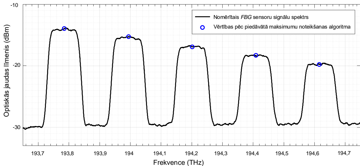
3.6. att. 5 FBG optisko sensoru atstaroto signālu amplitūdas frekvenču pārvades raksturlīknes spektrs ar precīzi noteiktām centrālām maksimumu frekvencēm izmantojot autora piedāvāto algoritmu.
