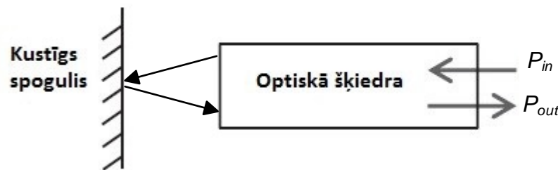
1.4. att. Vienkārša ārēja (angļu val. extrinsic ) intensitātes modulēta sensora uzbūve [104].
