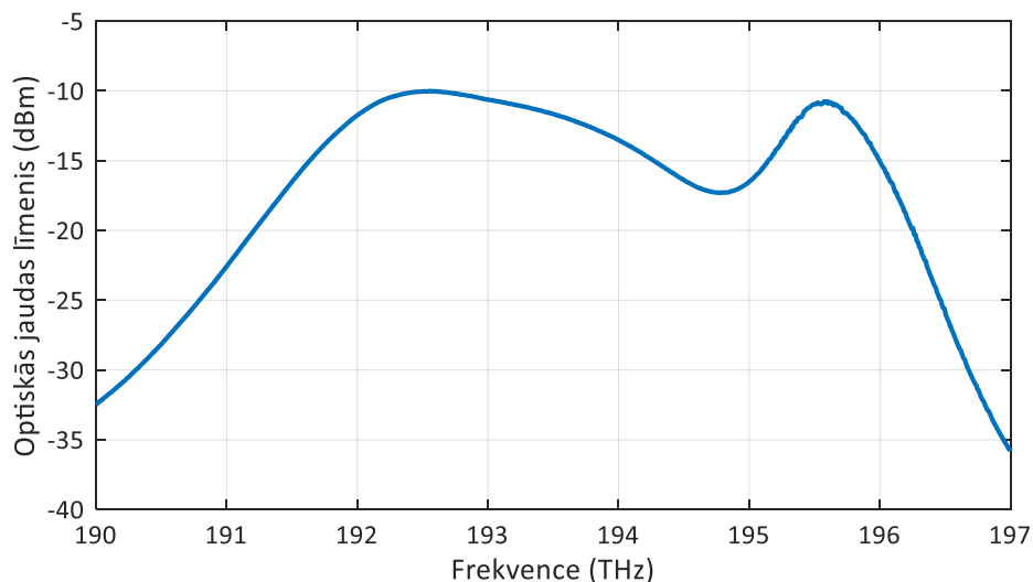
4.6. att. Platjoslas ASE gaismas avota eksperimentāli uzņemtais optiskais amplitūdas frekvenču pārvades raksturlīknes spektrs.
