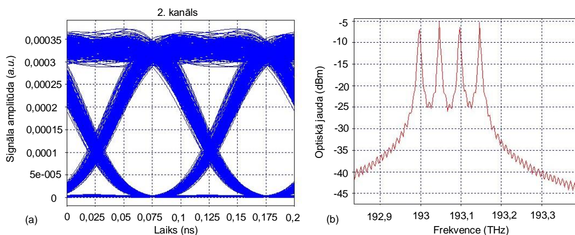
2.4. att. (a) uztvertā signāla acs diagramma (2. kanāls) pēc 20\text{ km} garas pārraides līnijas un (b) blīvas 10\text{ Gbit/s NRZ-OOK DWDM} pārraides sistēmas pārraidītais amplitūdas frekvenču pārvades raksturlīknes spektrs ar 50\text{ GHz} starpkanālu intervālu.
