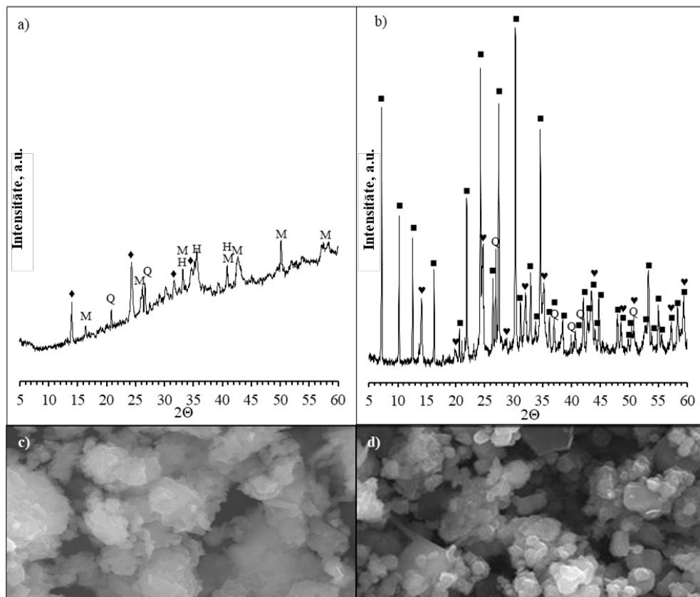
4.1. att. Sintēze ceļā no elektrofiltru pelniem iegūtais ceolīta C1 un no metakaoļina iegūtais ceolīts C2; a) C1 rentgenstaru difraktogramma, Q – kvarcs (85–0335), M – mullīts (83–1881), H – hematīts (72–0469), ♦ – ceolīts P1 (84–0698); b) C2 rentgenstaru difraktogramma, Q – kvarcs (85–0335), ■ – ceolīts A (39–0222), ♥ – hidroksilsodalīts (11–0401); c) C1 mikrostruktūra, palielinājums 10000 reizes; d) C2 mikrostruktūra, palielinājums 3000 reizes.
