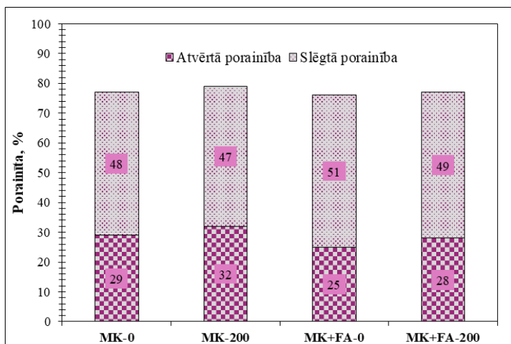
4.21. att. Porainu ģeopolimēru porainība.
