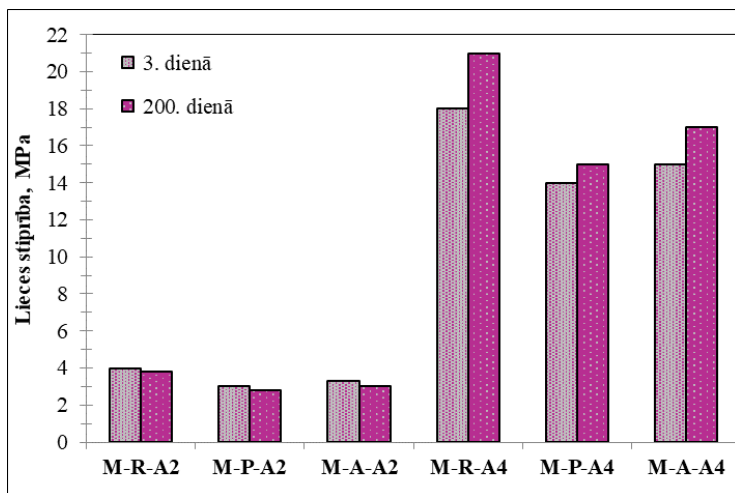
4.32. att. Izgatavoto ģeopolimēru saistvielu lieces stiprība.
