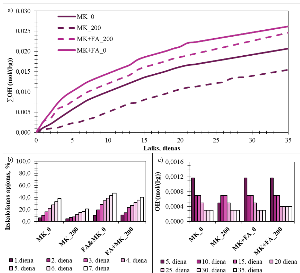
4.29. att. a) \text{OH}^- jonu kumulatīvais izskalošanās ātrums; b) \text{OH}^- jonu izskalošanās pirmajā testa nedēļā salīdzinājumā ar kopējo izskalo to \text{OH}^- jonu daudzumu 35 dienu laikā; c) kopējais \text{OH}^- daudzums ik katrās piecās testa dienās.
