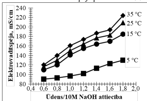
4.4. att. Aktivizācijas šķīduma koncentrācijas ietekme uz ģeopolimēra saistvielas elektrovadītspēju.
