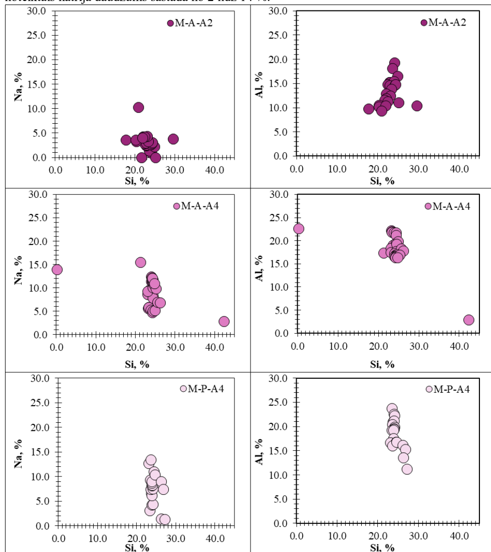
4.36. att. Ģeopolimēru saistvielas EDX analīze, katra apskatītā spektra punkta Na&Si un Al&Si procentuālais sadalījums.
