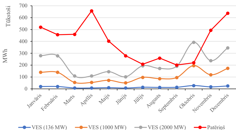
3.24. att. Vēja enerģijas ražošana (zilā līnija) un patēriņš (sarkanā līnija) Latvijā 2022. gadā, vēja enerģijas ražošana, ja jauda būtu 1000 MW (zaļā līnija) un ja jauda būtu 2000 MW (pelēkā līnija).
